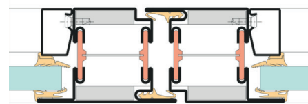
Coupe de détails de la porte coupe feu
