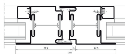
Coupe de détails PA60_Élégance
