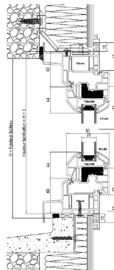
Isolation intérieure de 100 mm (possible de 70 à 180 mm)
