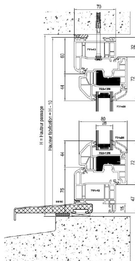
Pièce d'appui de 100 mm en base (possible en 70 et 123 mm)
