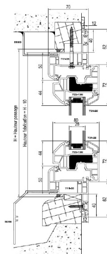
Ailette rénovation de 40 mm en base (possible en aile de 27 et 60 mm en blanc)
